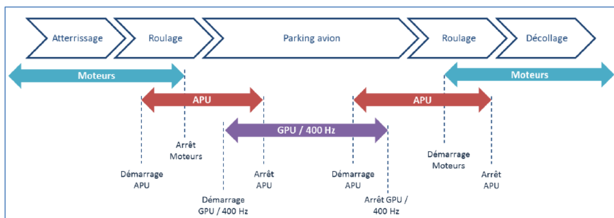
Figure 14 - Utilisation des auxiliaires de puissance durant une escale - Source : I Care & Consult 35
